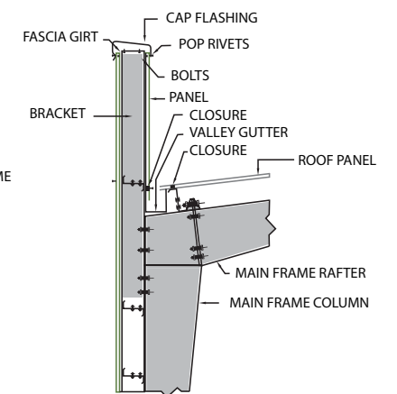
Parapet Fascia
